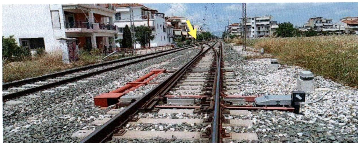
ΕΙΚΟΝΑ 10 ΚΛΕΙΔΙ 118 Α. Μετάβαση από γραμμή ανόδου σε γραμμή καθόδου. Στο βάθος αριστερά το 118 Β ( κίτρινο βέλος).
